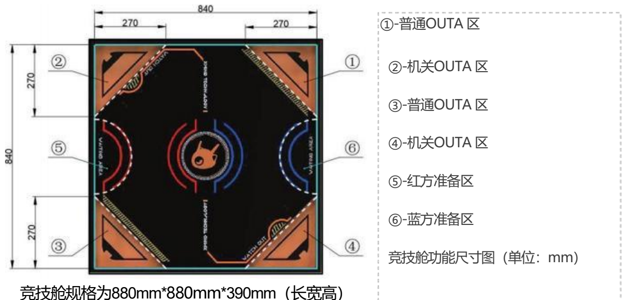
竞赛场地俯视渲染图竞赛场地渲染图
