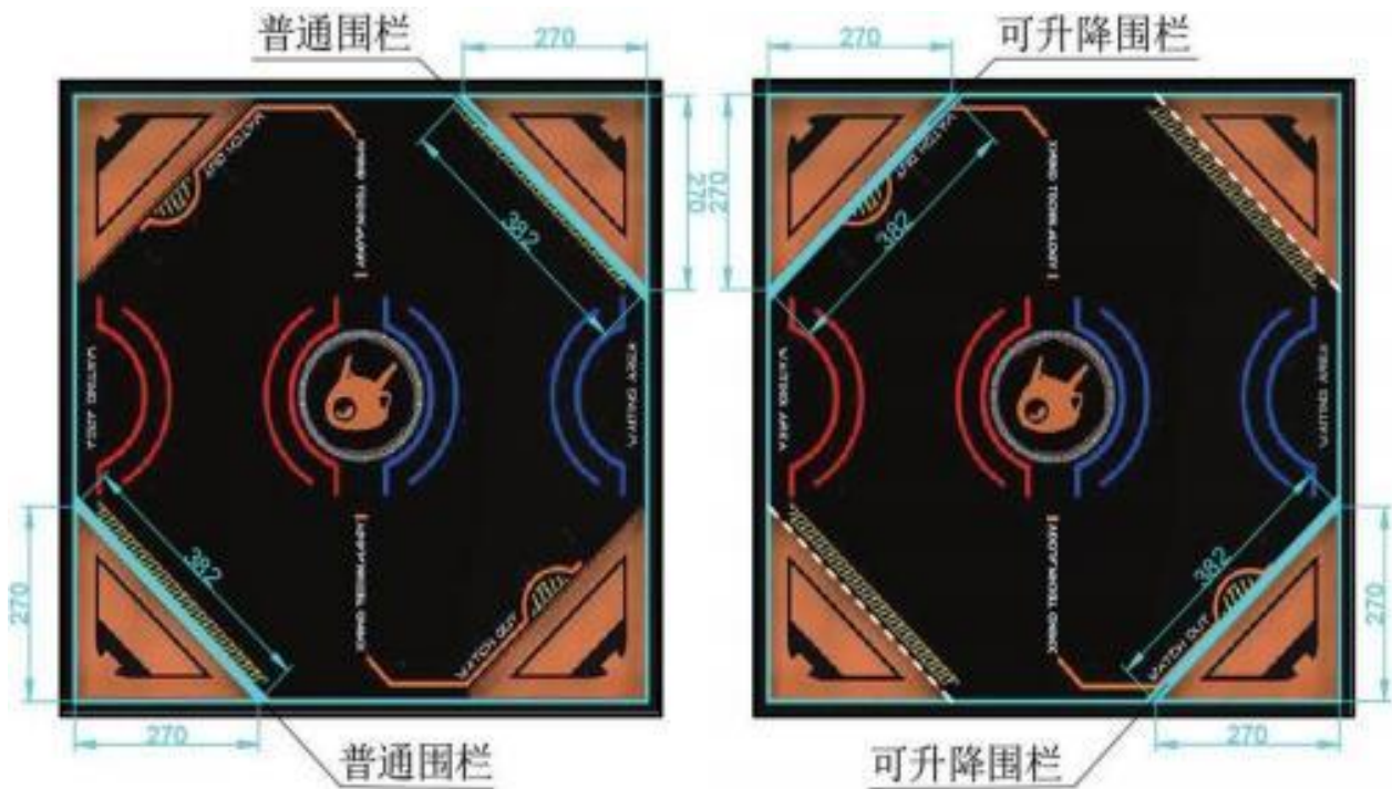
普通OUTA区示意图 机关OUTA区示意图
