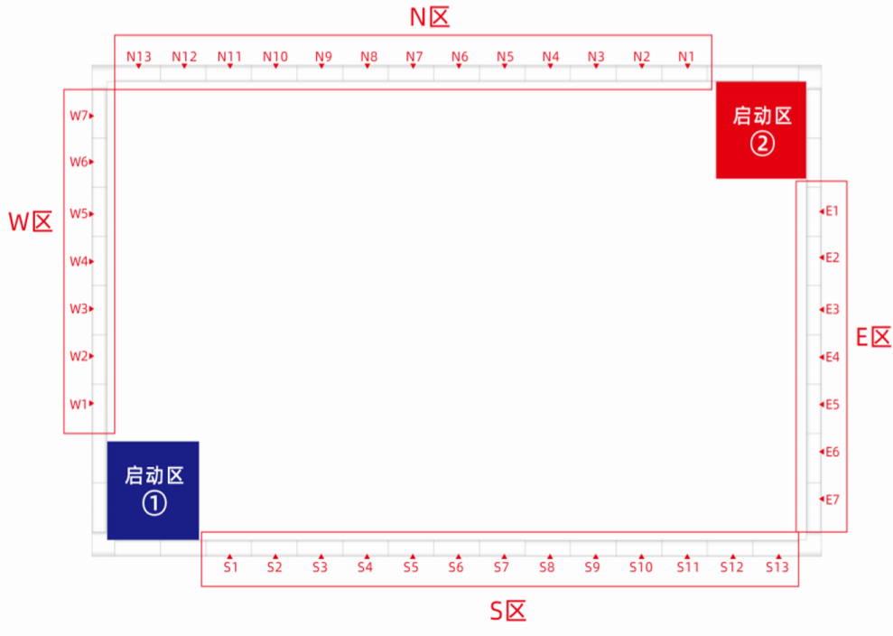
图 11 赛台围栏分区及编号
